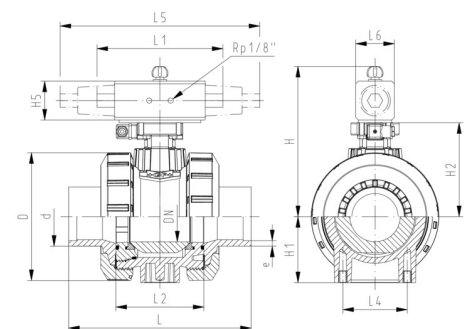
DN65-100
