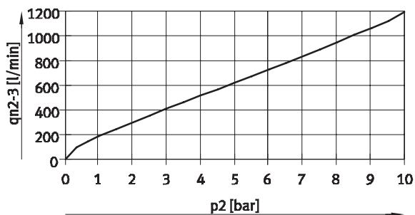
VPPM-6TA-...-0L10H-... (10 bar)
