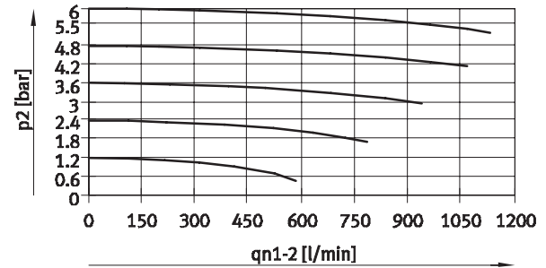
VPPM-6TA-...-0L6H-... (6 bar)
