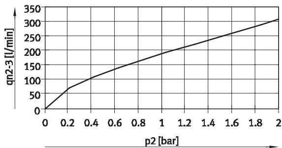
VPPM-6TA-...-0L2H-... (2 bar)
