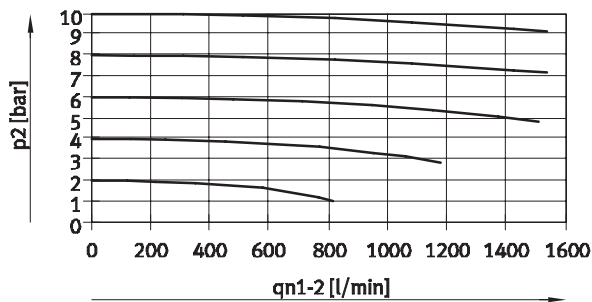
VPPM-6TA-...-0L10H-... (10 bar)
