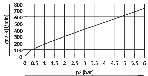
VPPM-6TA-...-0L6H-... (6 bar)
