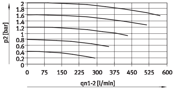
VPPM-6TA-...-0L2H-... (2 bar)
