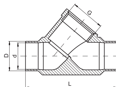
"M"- Anschweißenden DIN 11850-R2
