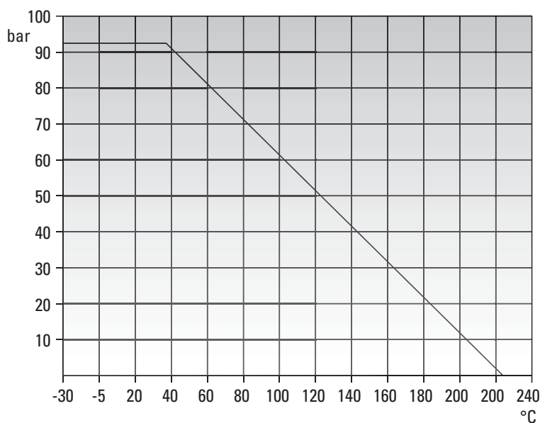
Druck-Temperatur-Diagramm (PTFE-glasfaserverstärkt) / Pressure-Temperature-Diagram (PTFE glassfiber reinforced)
