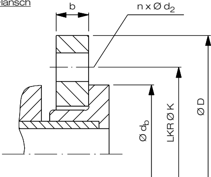
Flansch
