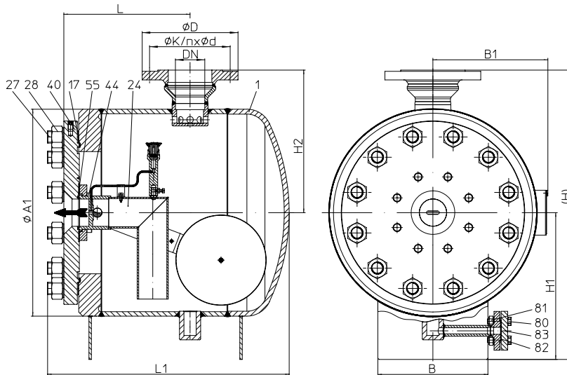
Fig. 638....1 ECK-Ausführung mit Flanschen (Zulauf von oben)
