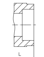
Fig. 630...3 mit Schweißmuffen
