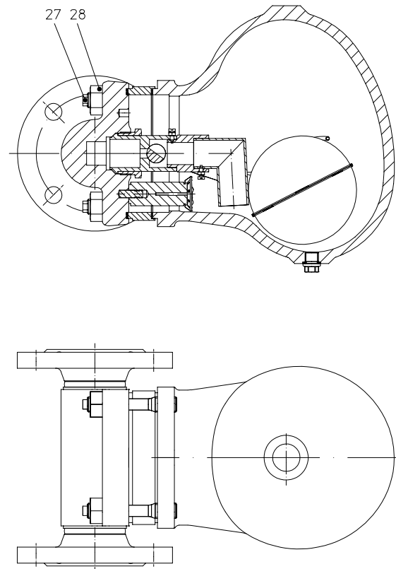
Fig. 633....1 mit Flanschen - horizontale Einbaulage
