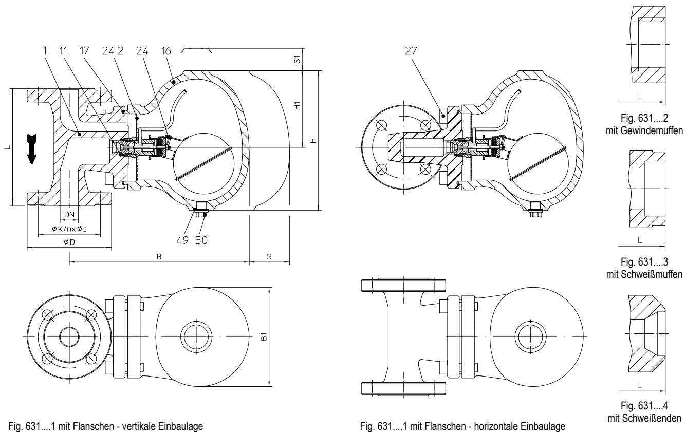
Fig. 631....1 mit Flanschen - vertikale Einbaulage
