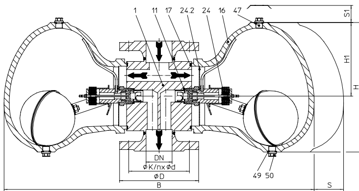
Fig. 639....1 mit Flanschen - vertikale Einbaulage
