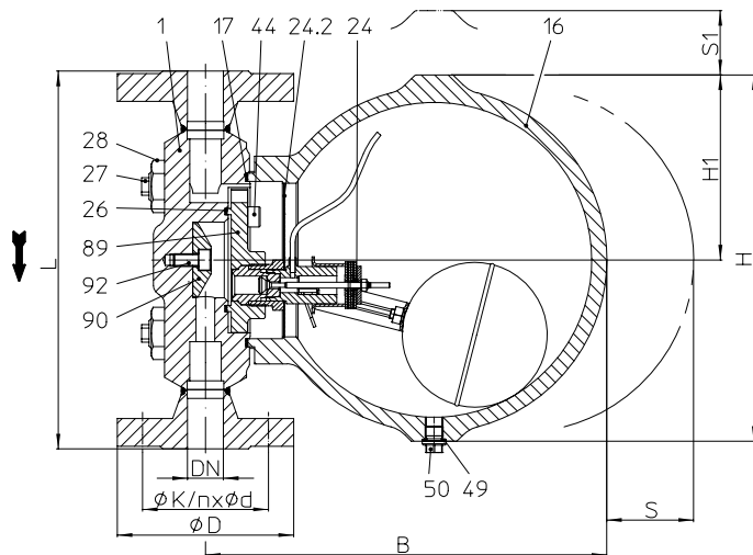
Fig. 631...1 mit Flanschen - vertikale Einbaulage (PN100)
