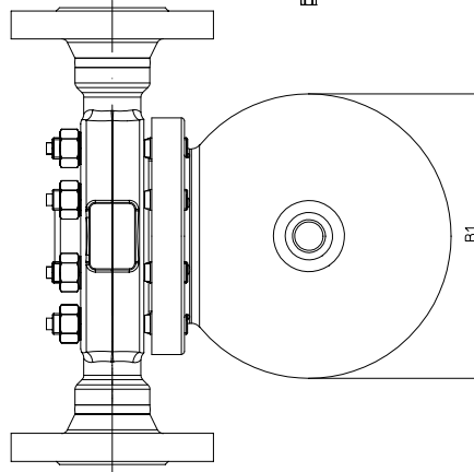
Fig. 631...1 Durchgangs-Ausführung mit Flanschen - horizontale Einbaulage
