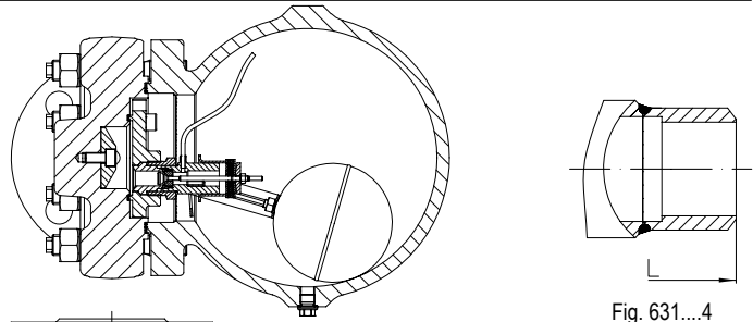
Fig. 631...4 mit Schweißenden
