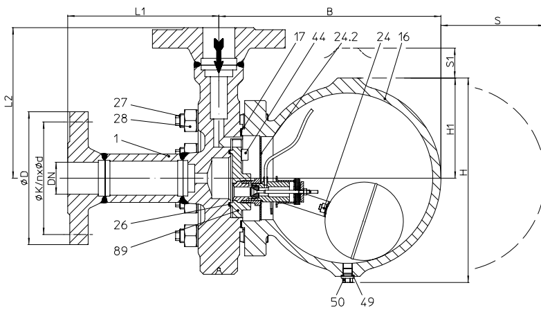
Fig. 632...1 ECK-Ausführung mit Flanschen - vertikale Einbaulage
