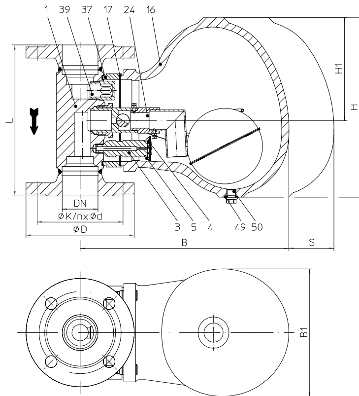
Fig. 633....1 mit Flanschen - vertikale Einbaulage
