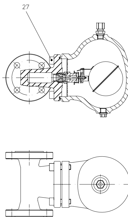
Fig. 630...1 mit Flanschen - horizontale Einbaulage
