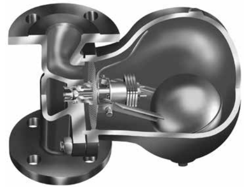
Fig. 631....1 vertikale Einbaulage
