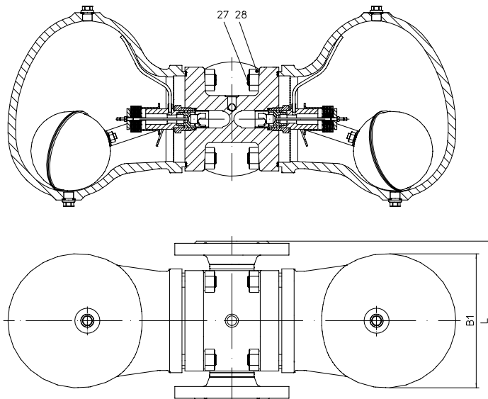
Fig. 639....1 mit Flanschen - horizontale Einbaulage
